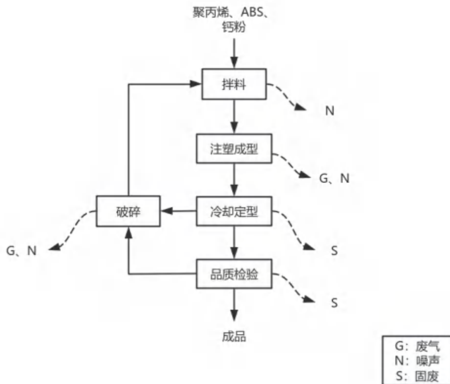
图 2-1 注塑区域工艺流程及产污环节图
